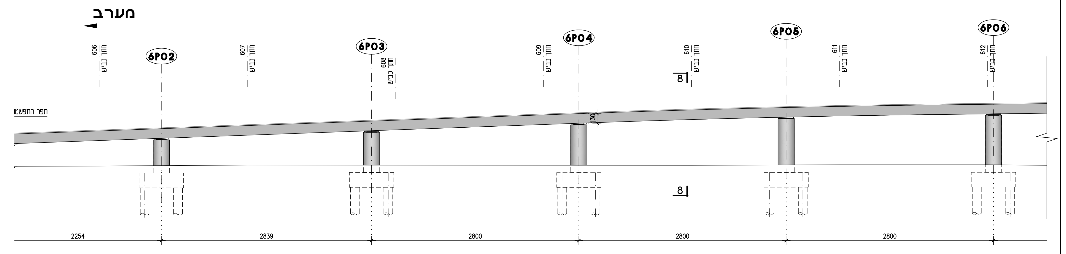
חתר לאורך ציר 6 (קטע מערבי) 1:250
