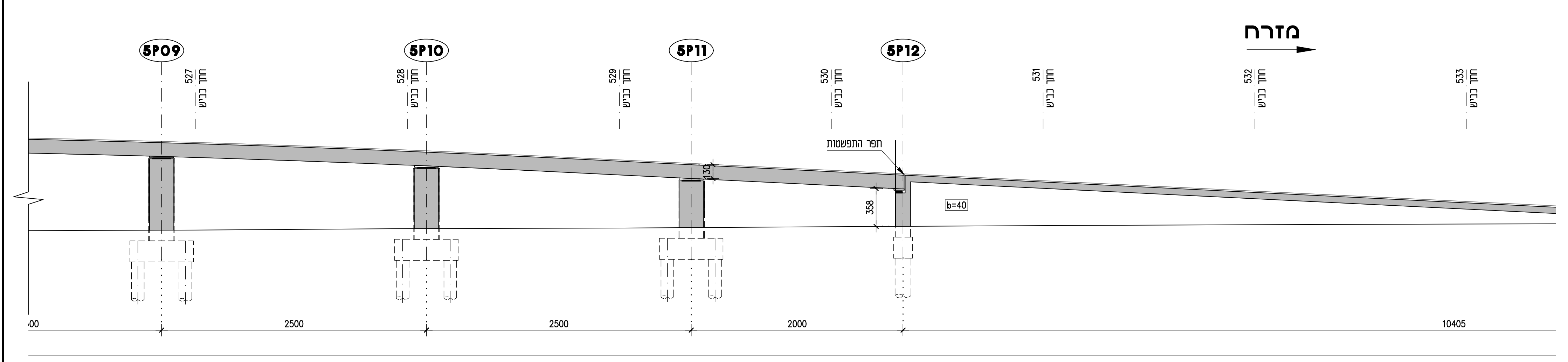
חתר לאורך ציר 5 - דרך אם המושבות (קטע מזרחי) 1:250
