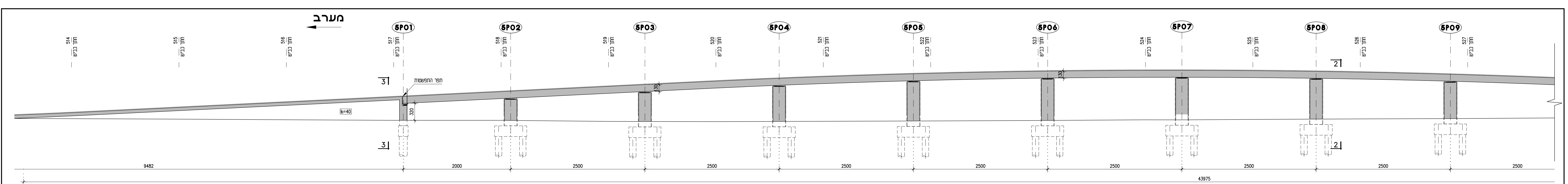
חתר לאורך ציר 5 - דרך אם המושבות (קטע מערבי) 1:250
