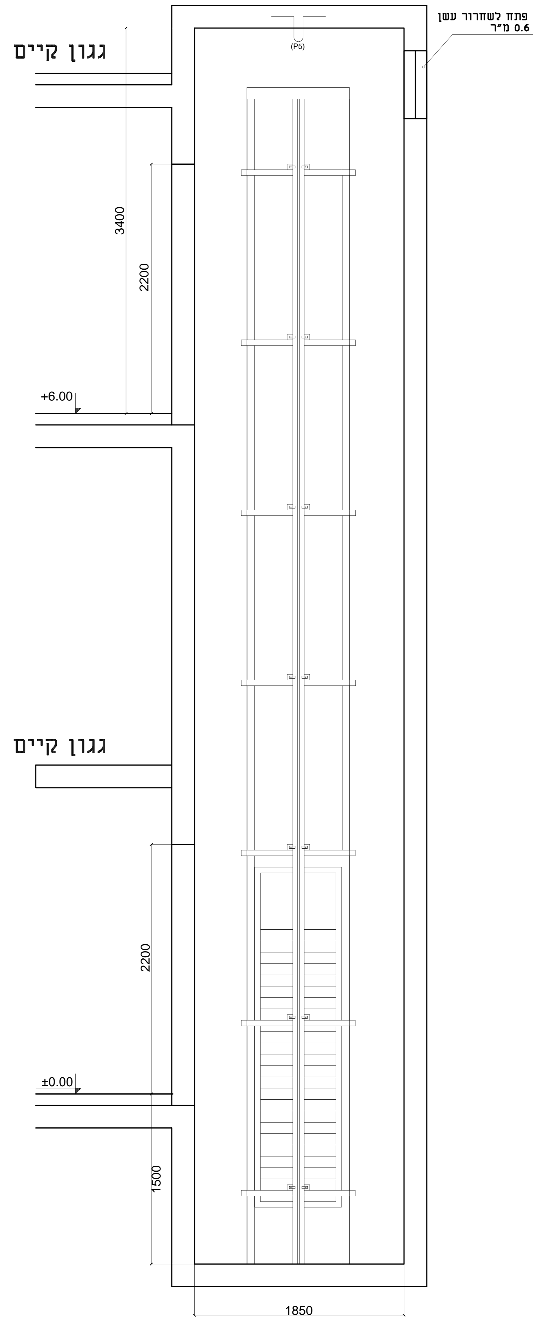
חתך - בניה א - א
