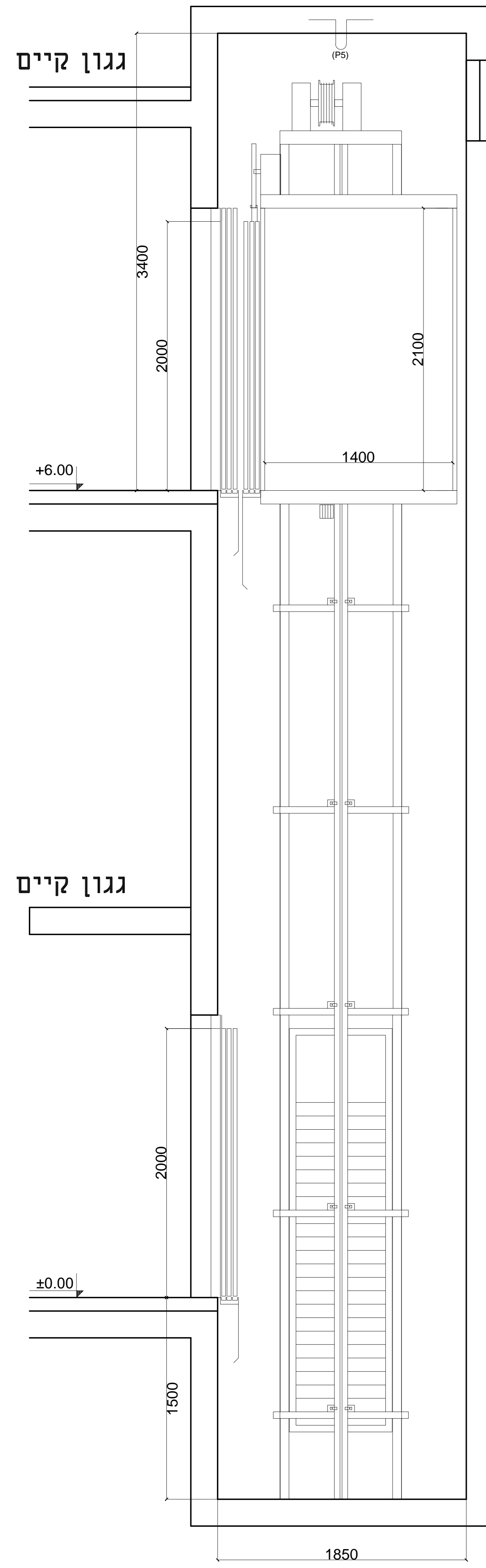
חתך - כללי א - א
