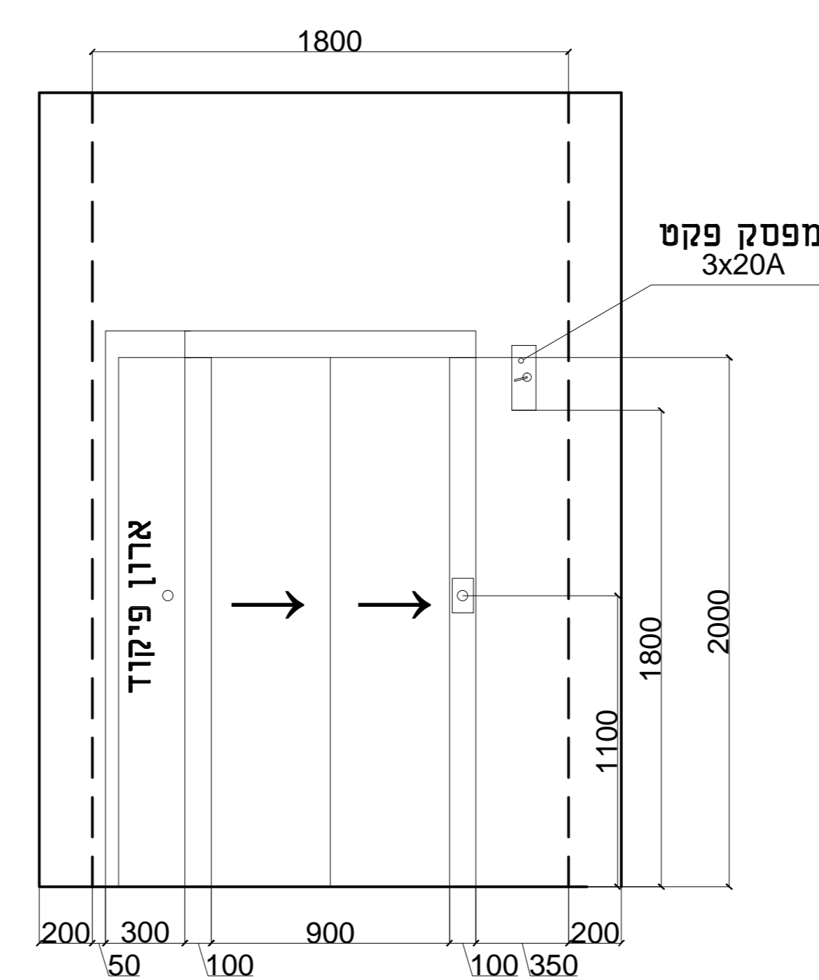
חזית - כללי תחנה עליונה בלבד
