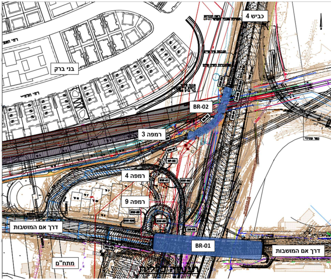
תרשים גבולות תימרור סופיים (רשות תימרור נת"י - ורוד)
